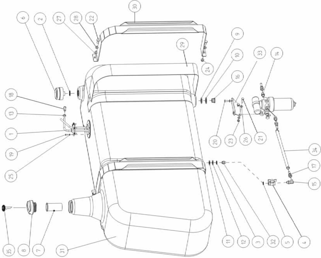
Kraftstofftank 350 3A Fuel tank 350 3A
